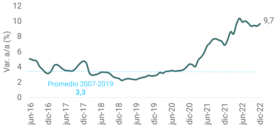
Gráfico 5. Crecimiento de costos de construcción de vivienda
