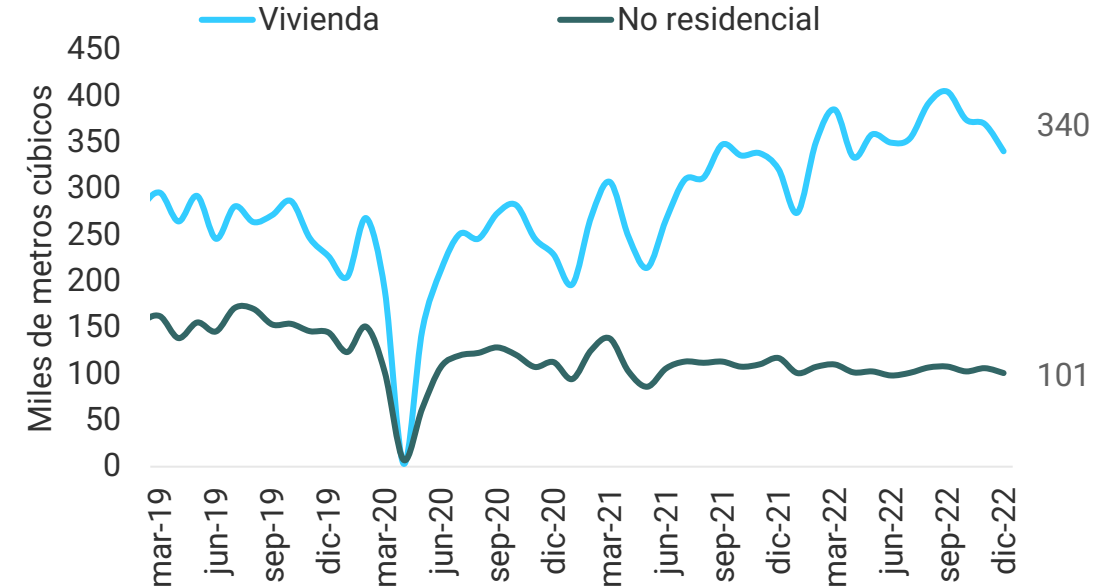
Gráfico 4. Concreto premezclado por destino
